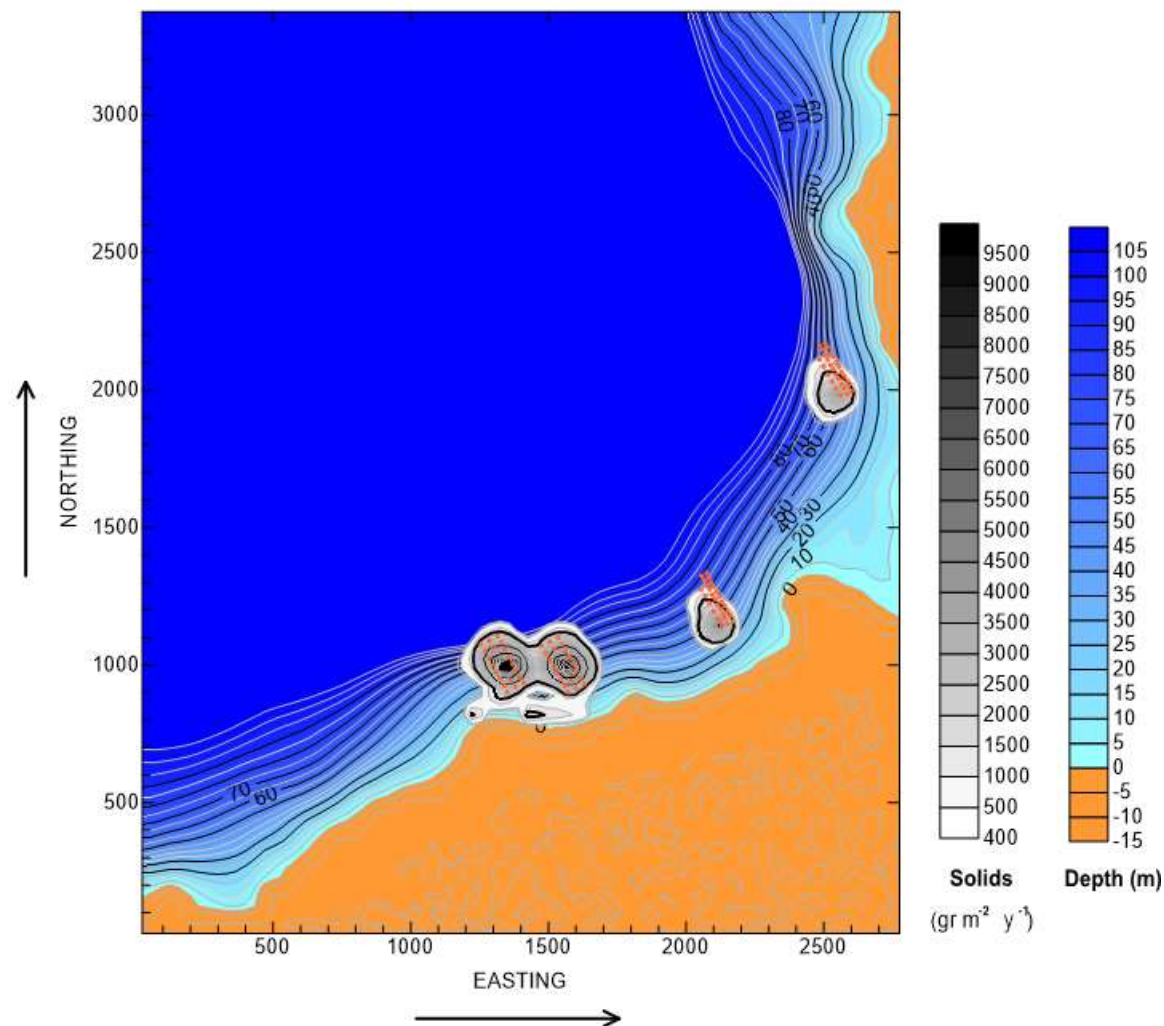
Εικόνα 7.1 Εκτίμηση διασποράς στερεών αποβλήτων (Πόρος – Σενάριο1).
