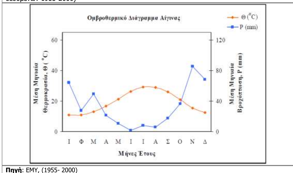
Εικόνα 6.3 Ομβροθερμικό Διάγραμμα για τον μετεωρολογικό σταθμό της Αίγινας (περίοδος δεδομένων 1955-2000)
