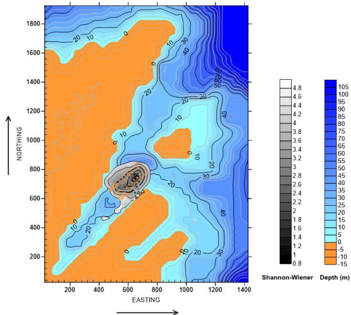
Εικόνα 7.5 Μεταβολή ποικιλότητας βενθικής κοινωνίας (Μπίστι – Σενάριο1).
