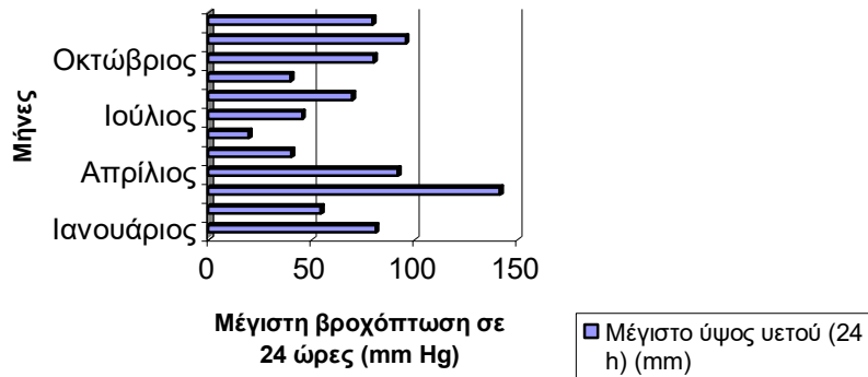
Εικόνα 6.5: Ραβδόγραμμα μέγιστων βροχοπτώσεων.
