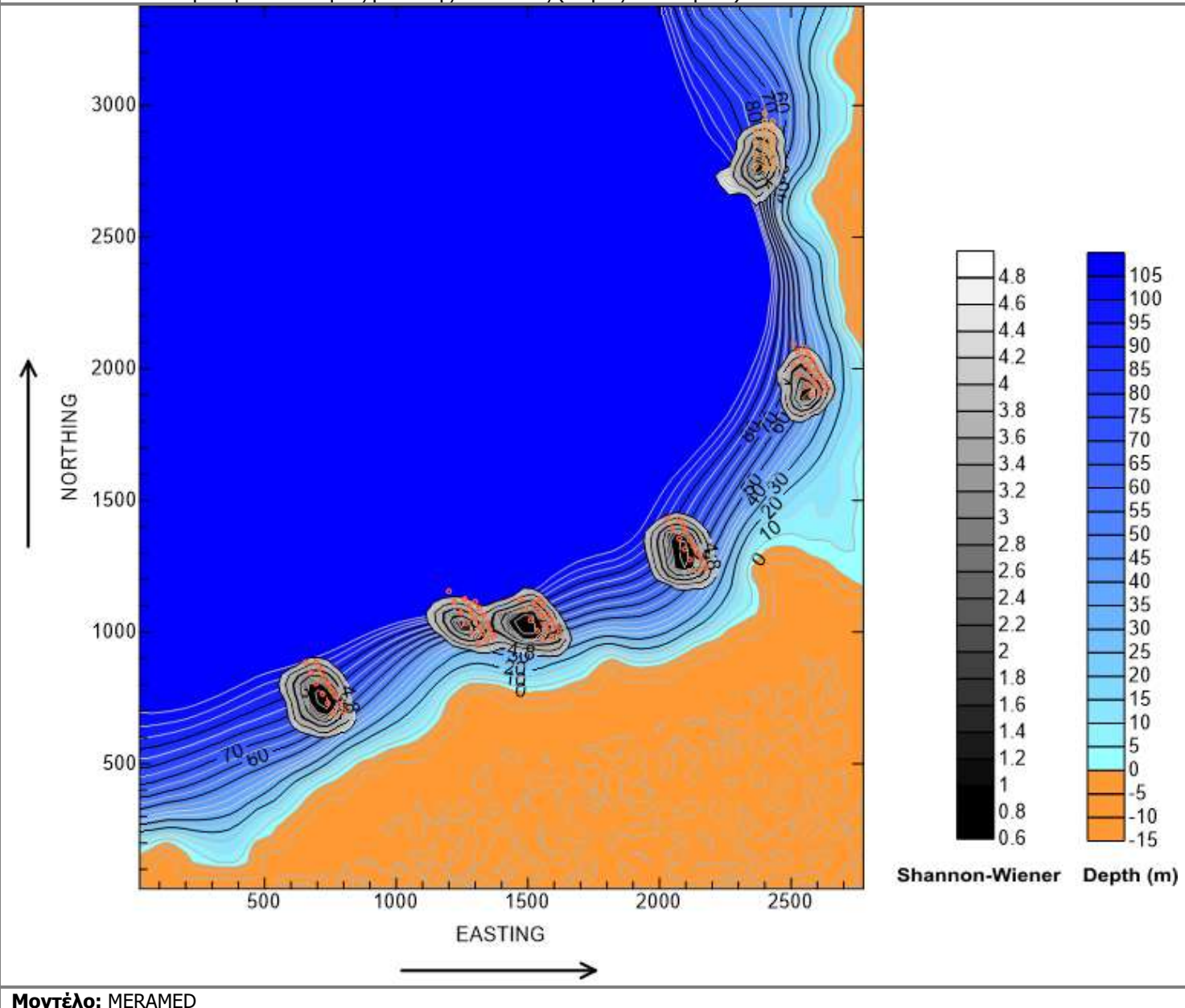
Εικόνα 7.17 Μεταβολή ποικιλότητας βενθικής κοινωνίας (Πόρος – Σενάριο4).
