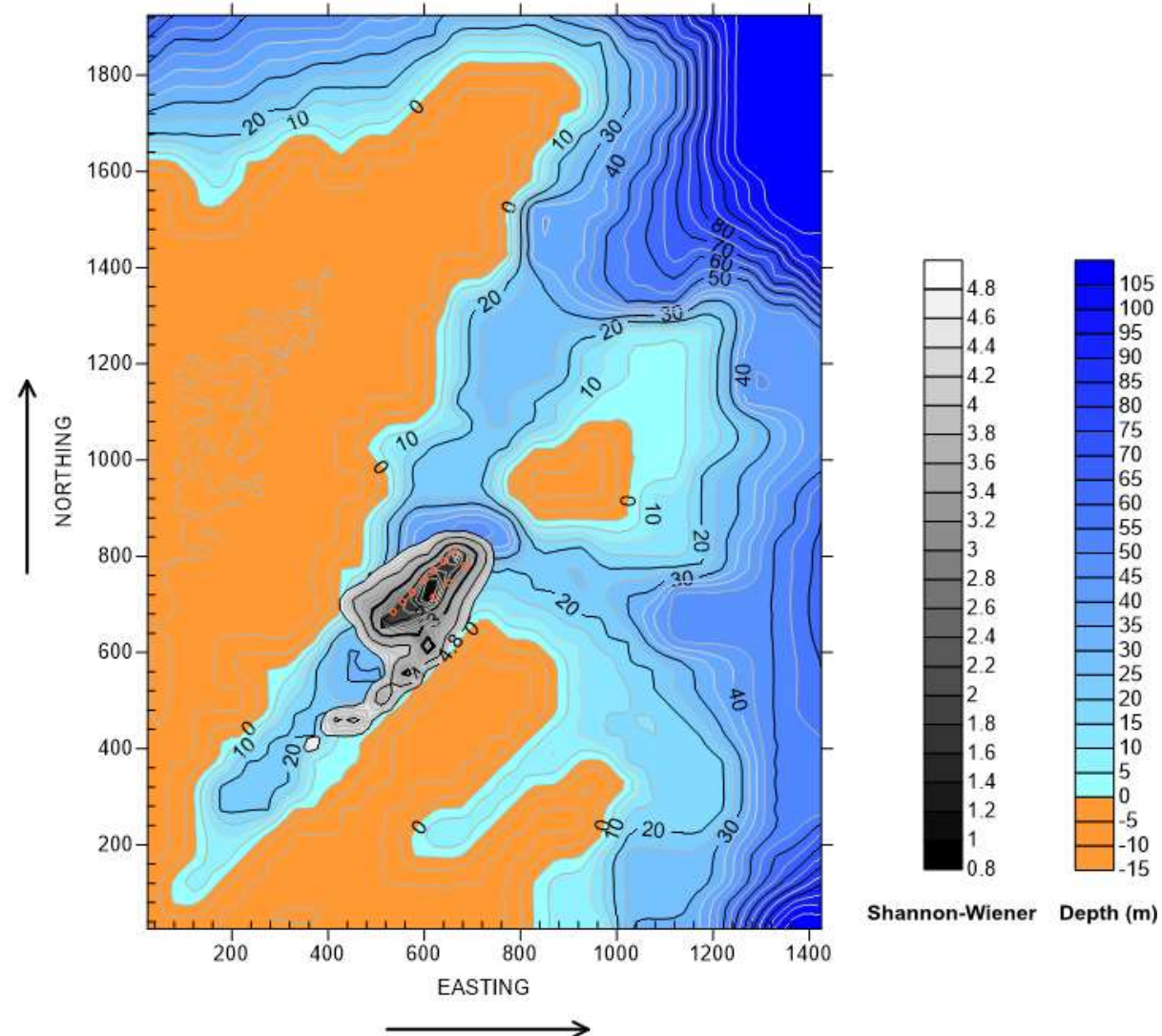
Εικόνα 7.11 Μεταβολή ποικιλότητας βενθικής κοινωνίας (Μπίστι – Σενάριο2).
