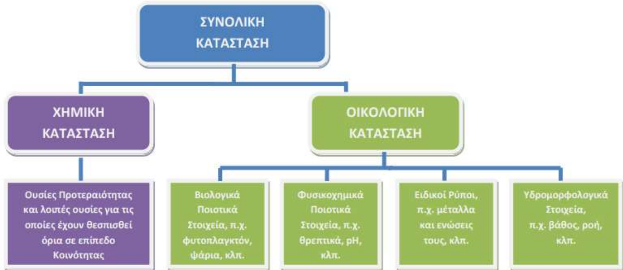
Διάγραμμα 6.1 Κατηγορίες ποιοτικών στοιχείων που χρησιμοποιούνται για την αξιολόγηση της κατάστασης των επιφανειακών υδατικών συστημάτων.
