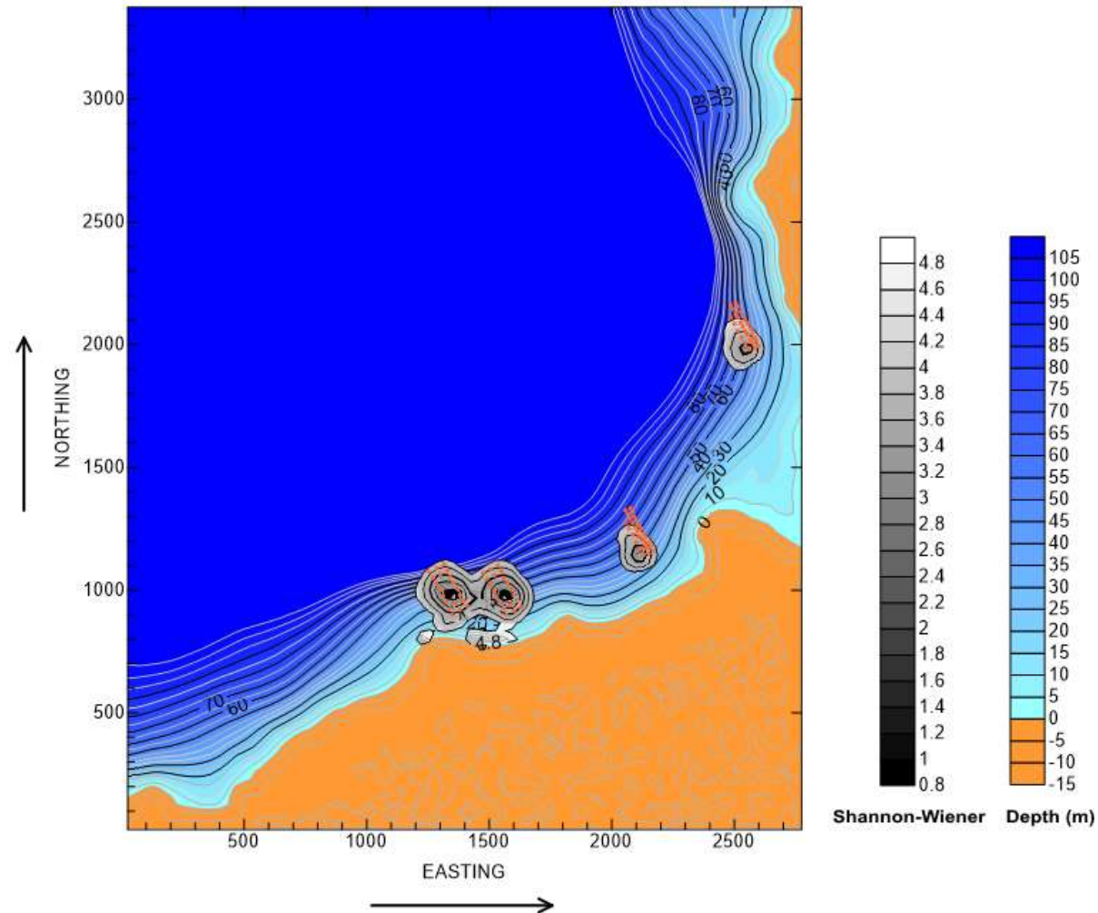
Εικόνα 7.2 Μεταβολή ποικιλότητας βενθικής κοινωνίας (Πόρος – Σενάριο1).
