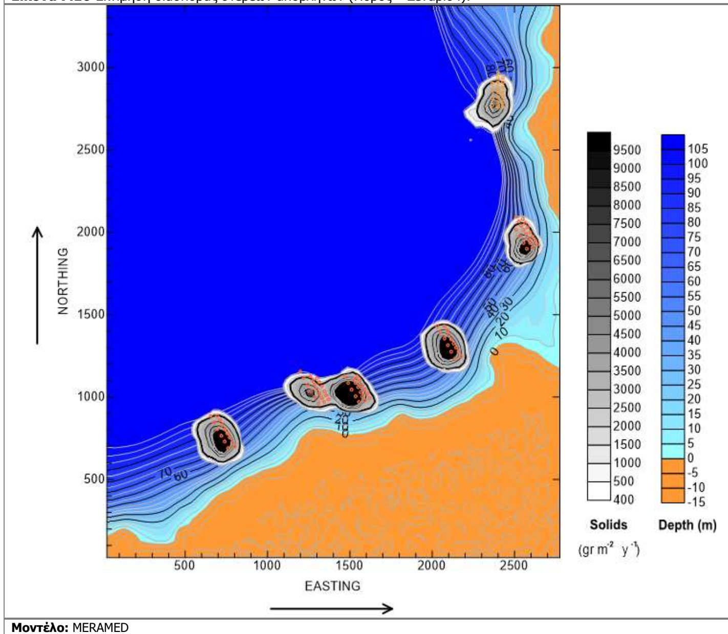
Εικόνα 7.16 Εκτίμηση διασποράς στερεών αποβλήτων (Πόρος – Σενάριο4).
