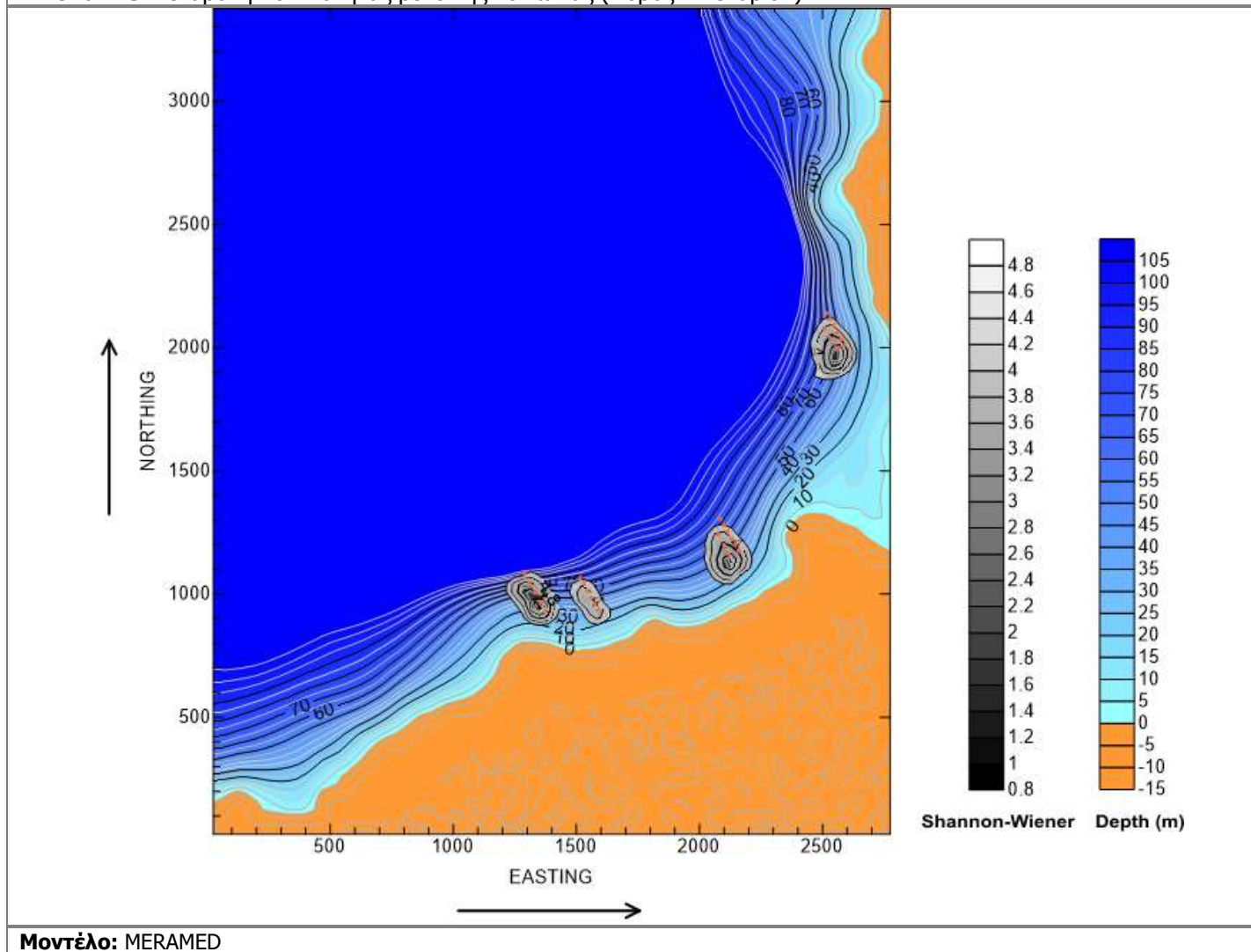
Εικόνα 7.8 Μεταβολή ποικιλότητας βενθικής κοινωνίας (Πόρος – Σενάριο2).
