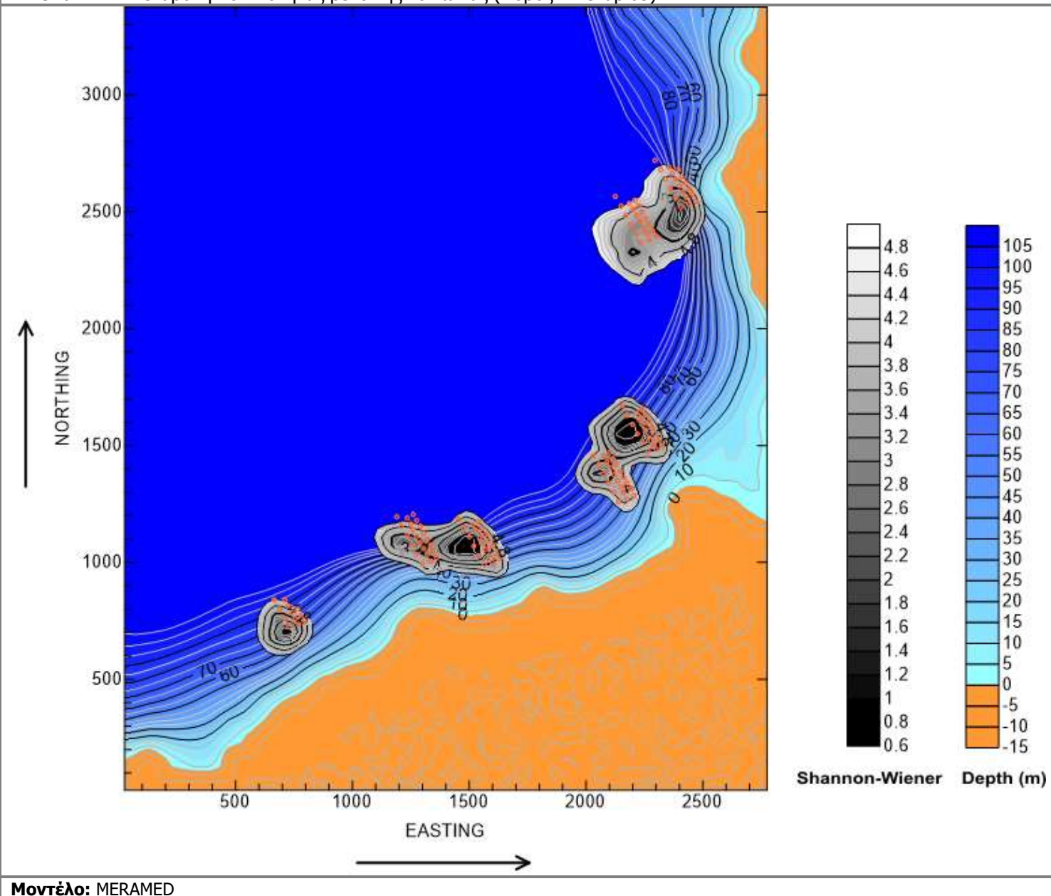
Εικόνα 7.14 Μεταβολή ποικιλότητας βενθικής κοινωνίας (Πόρος – Σενάριο3).
