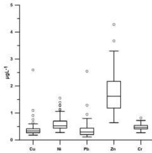
Εικόνα 6.1 Box-whisker διάγραμμα των συγκεντρώσεων Cu, Ni, Pb, Zn, Cr ( \mu\text{g L}^{-1} ).
