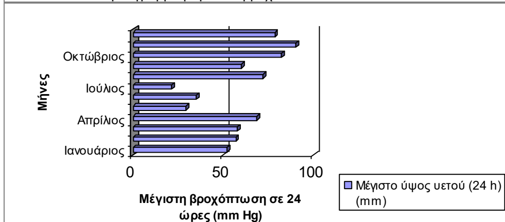
Εικόνα 6.10 Ραβδόγραμμα μεγίστων βροχοπτώσεων.
