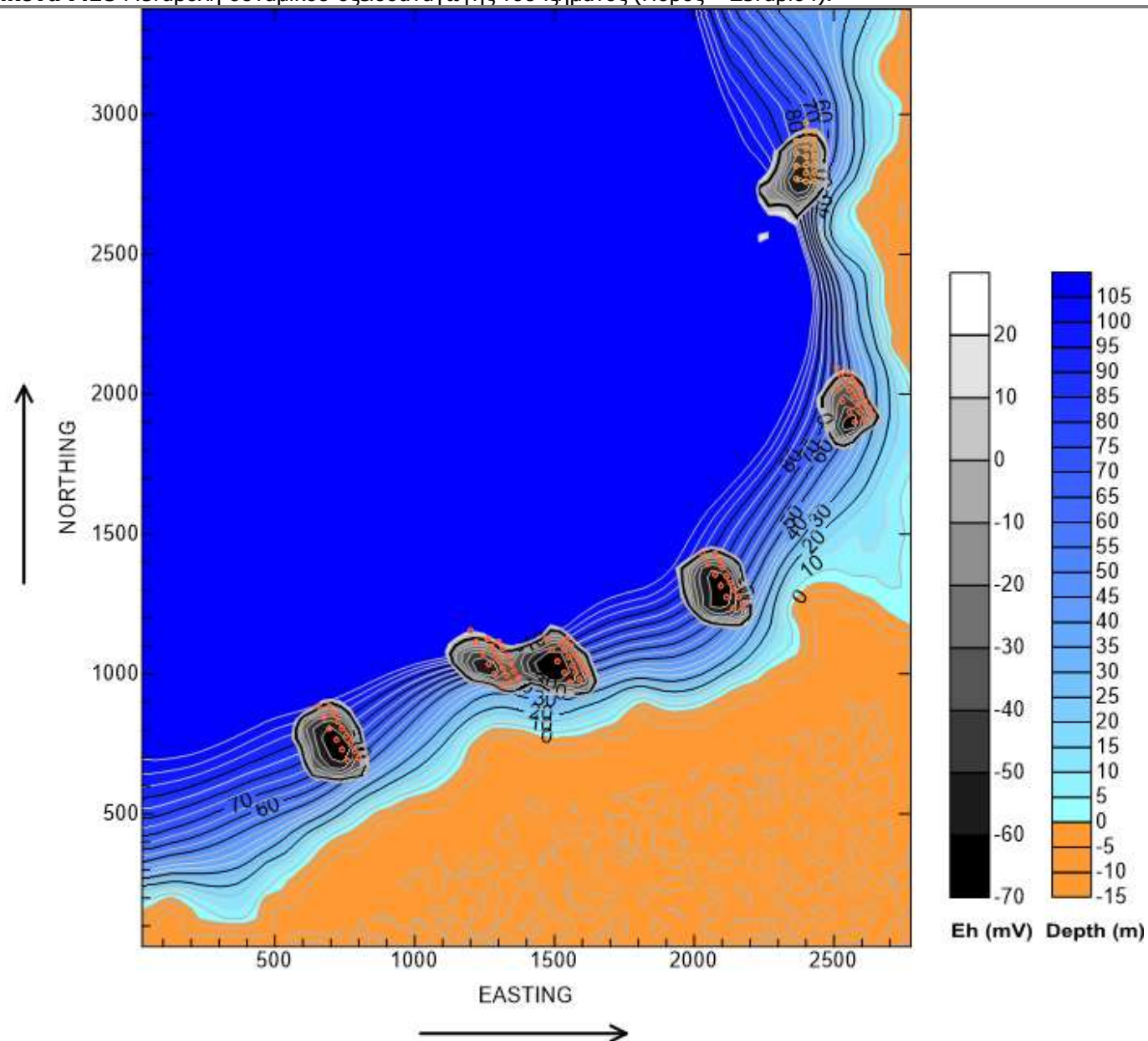
Εικόνα 7.18 Μεταβολή δυναμικού οξειδοαναγωγής του ιζήματος (Πόρος – Σενάριο4).
