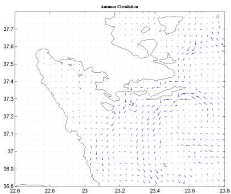
Εικόνα 6.15 Επικρατέστερες διευθύνσεις & ταχύτητες ρευμάτων το μήνα Οκτώβριο.
