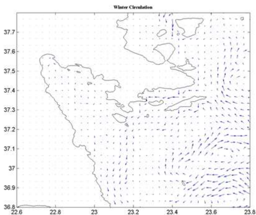
Εικόνα 6.12 Επικρατέστερες διευθύνσεις & ταχύτητες ρευμάτων το μήνα Ιανουάριο.
